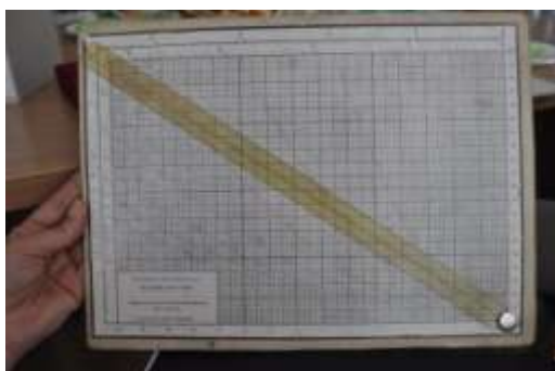
Nomogram tachimetryczny
